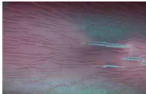
写真 4 CPVC 管のソルベントクラック
